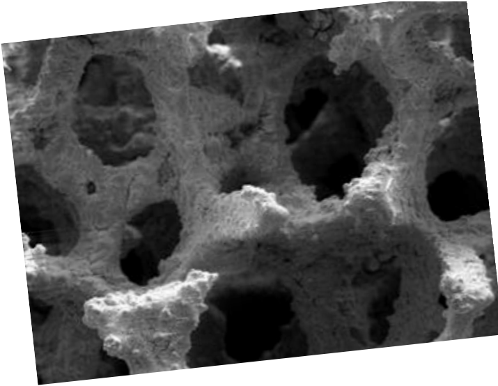
발포금속에 적용된 SEM 100X Catalyst
